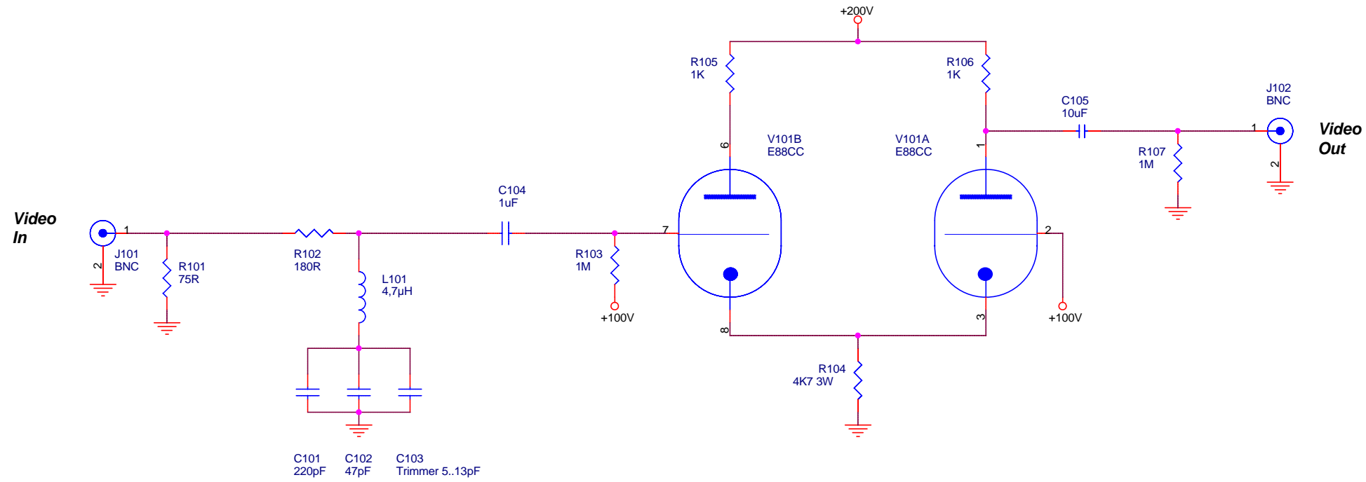
Notchfilter 4,43 MHz (Farbträger)
