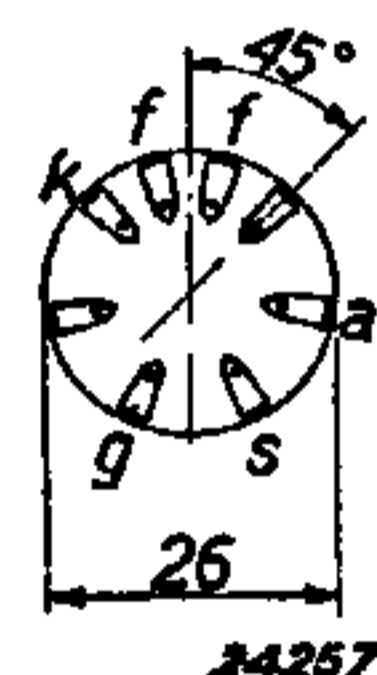
Abb. 2 Elektrodenanordnung und Sockelanschlüsse.
