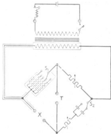
Bild 1 Schaltung der Meßbrücke
