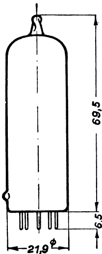
max. Abmessungen
