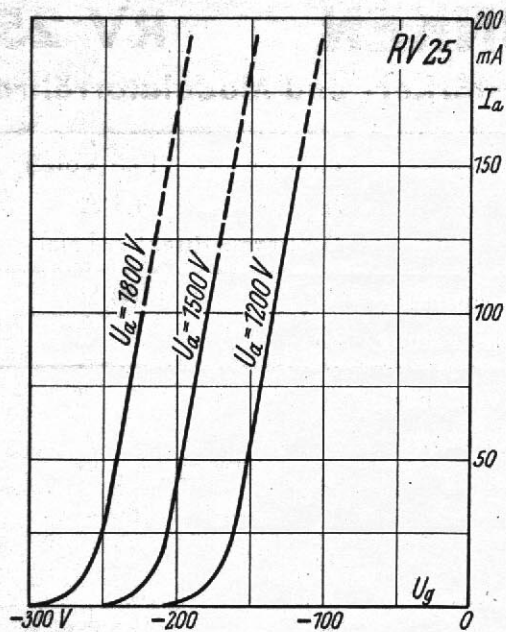
Statische Kennlinie der RV 25
