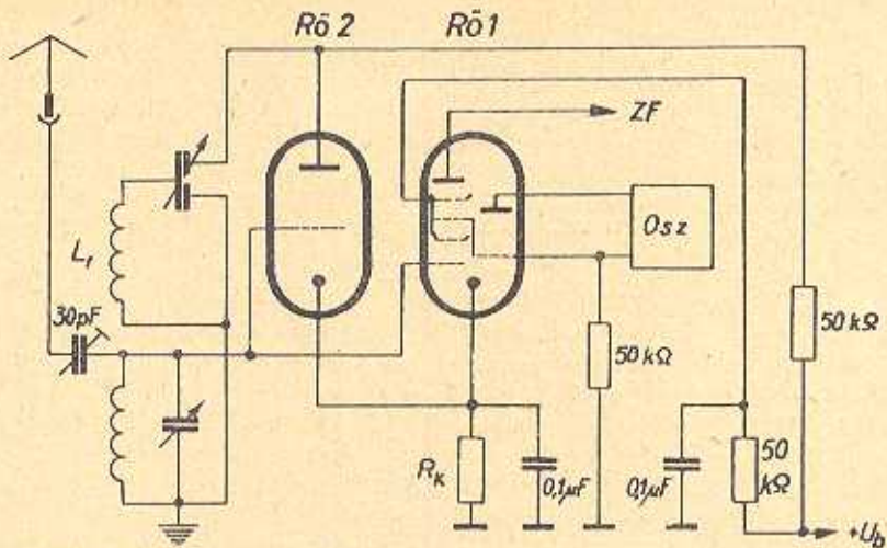
Abb. 119. HF-Entdämpfung des Eingangskreises mit einer getrennten Entdämpferöhre
