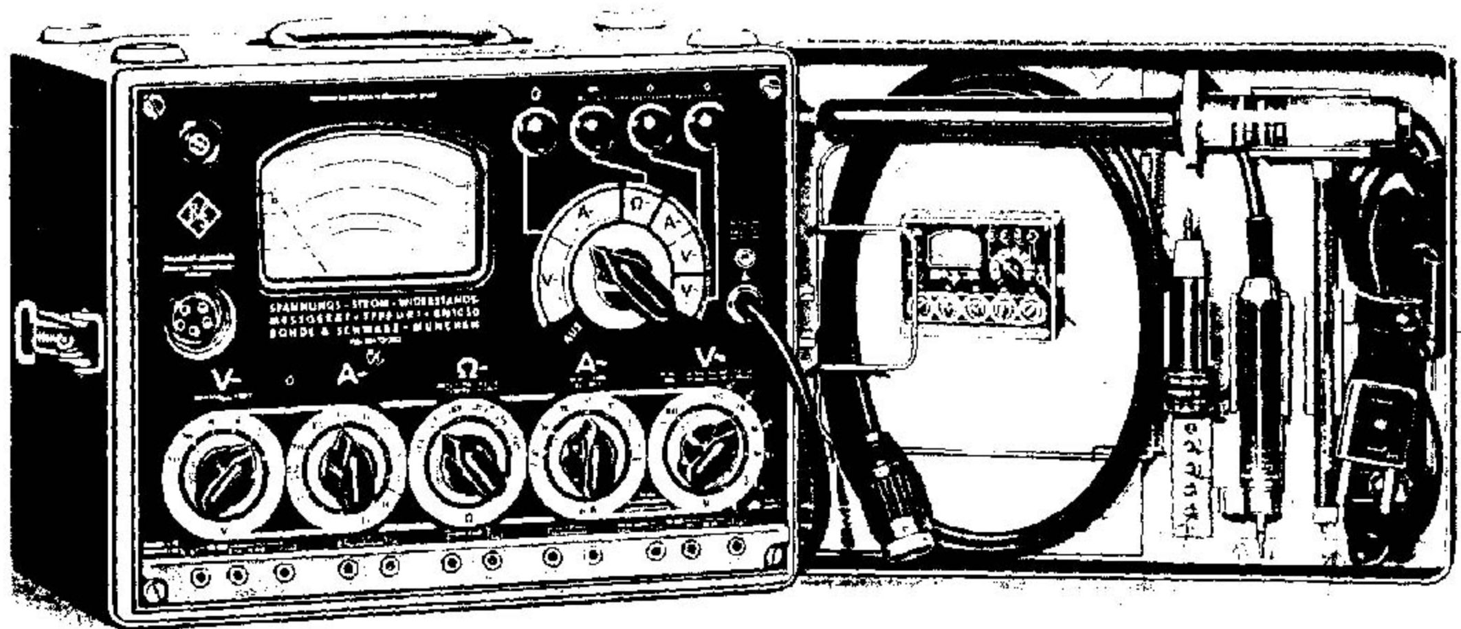
Bild 1 Spannungs-Strom-Widerstands-Meßgerät Type URI mit Zubehörteilen im Kastendecke!
