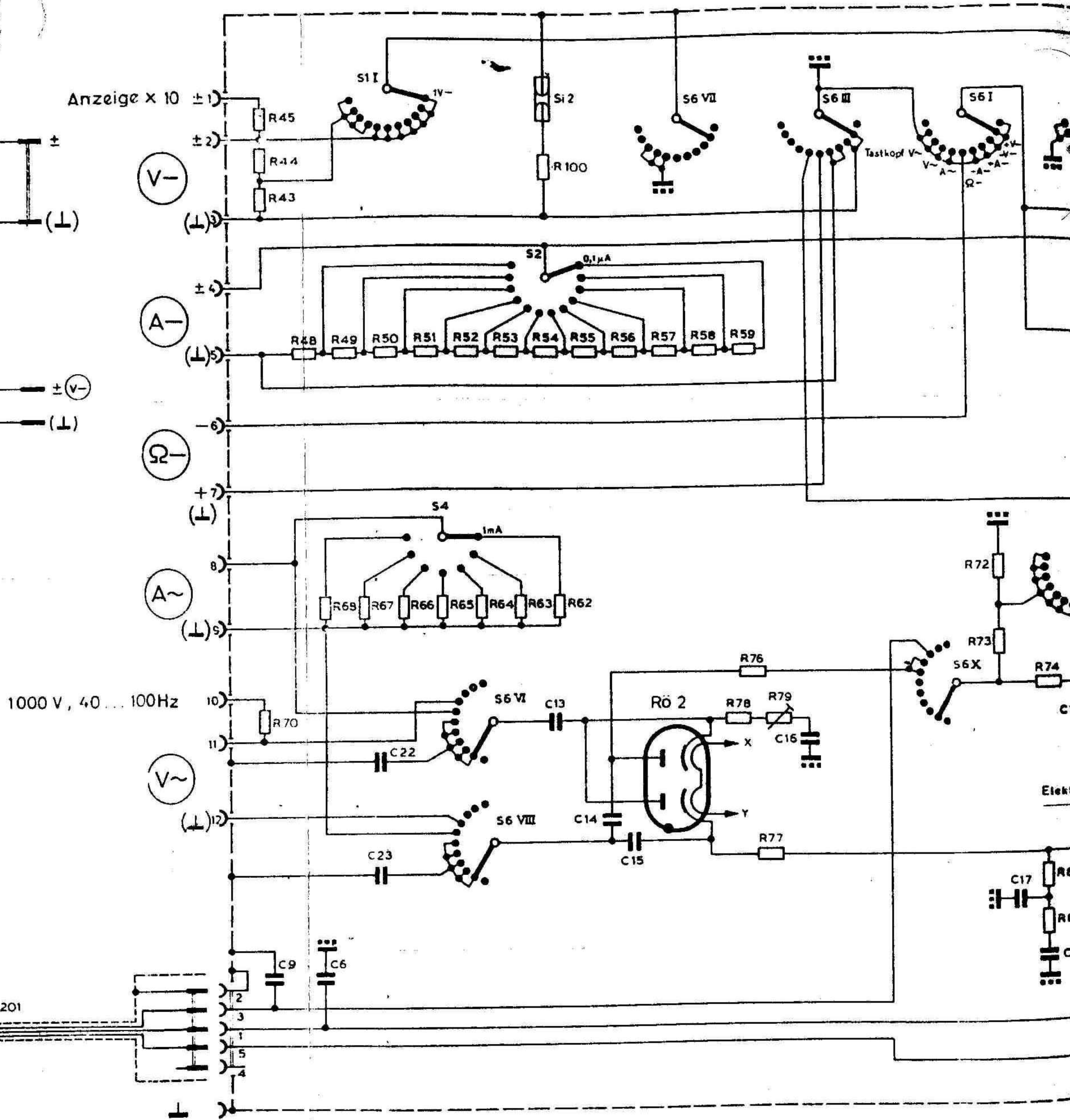
Bild 4. Stromlauf des Spannungs-Strom-Widerstands-Meßgerätes
